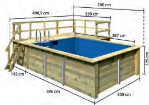
Maßangaben TREND HOLZPOOL 2 mit stirnseitiger und seitlicher Sonnenterrasse
