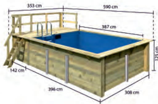
Maßangaben TREND HOLZPOOL 2 mit stirnseitiger Sonnenterrasse
