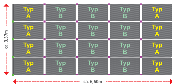
OKU Solarabsorber „Set 40“ Art. Nr. XXXXX
