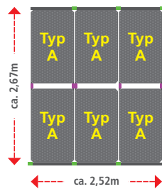
OKU Solarabsorber „Set 32b“ Art. Nr. XXXXX
