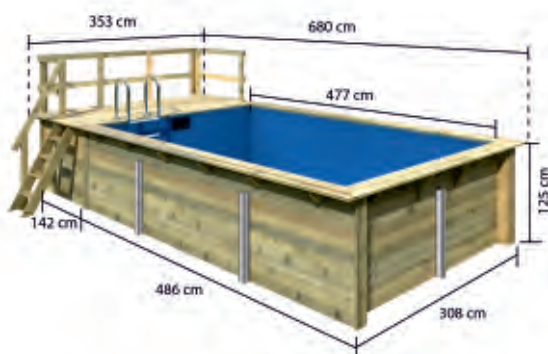
Maßangaben TREND HOLZPOOL 3 mit stirnseitiger Sonnenterrasse
