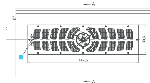
Unverbindliches Einbauschema
