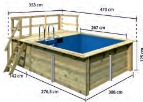
Maßangaben TREND HOLZPOOL 1 mit stirnseitiger Sonnenterrasse
