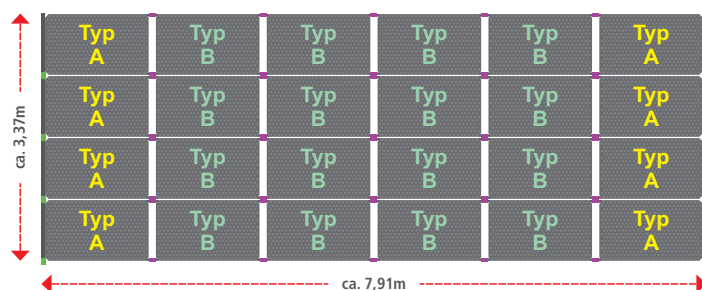
OKU Solarabsorber „Set 48“ Art. Nr. XXXXX
