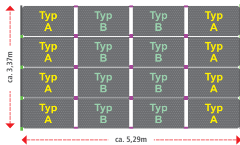
OKU Solarabsorber „Set 20a“ Art. Nr. XXXXX
