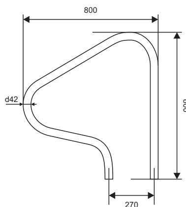
V2A Handlaufpaar Variante 1 Art-Nr. 52831-wp
