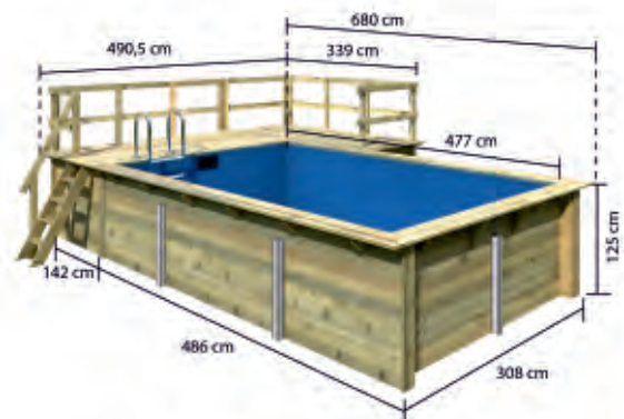
Maßangaben TREND HOLZPOOL 3 mit stirnseitiger und seitlicher Sonnenterrasse
