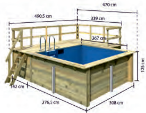
Maßangaben TREND HOLZPOOL 1 mit stirnseitiger und seitlicher Sonnenterrasse
