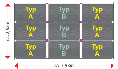
OKU Solarabsorber „Set 18“ Art. Nr. XXXXX
