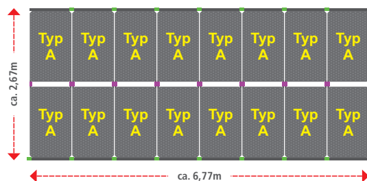
OKU Solarabsorber „Set 48“ Art. Nr. XXXXX
