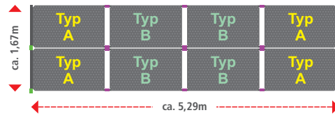
OKU Solarabsorber „Set 20b“ Art. Nr. XXXXX
