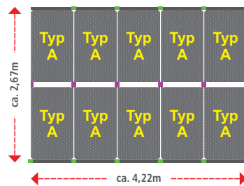
OKU Solarabsorber „Set 16b“ Art. Nr. XXXXX
